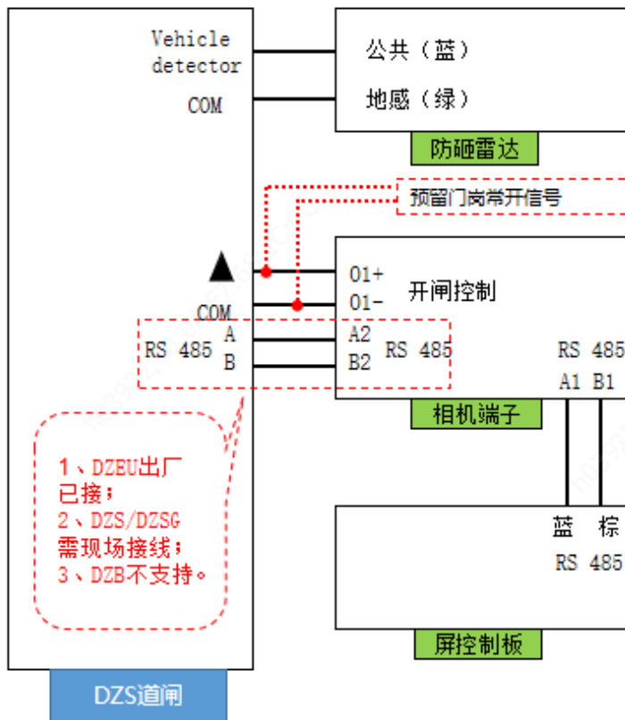
图6-2 整体接线示意图
