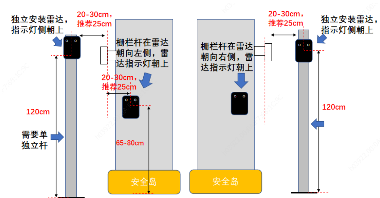
图4-4 安装示意图
