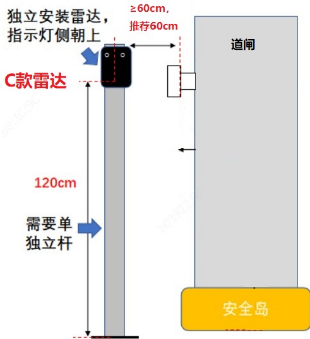
图5-4 C款雷达安装方案示意图
