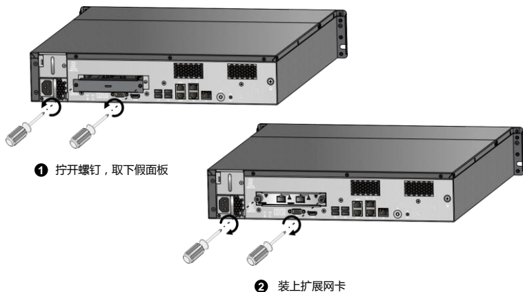
图2-5 安装扩展网卡
